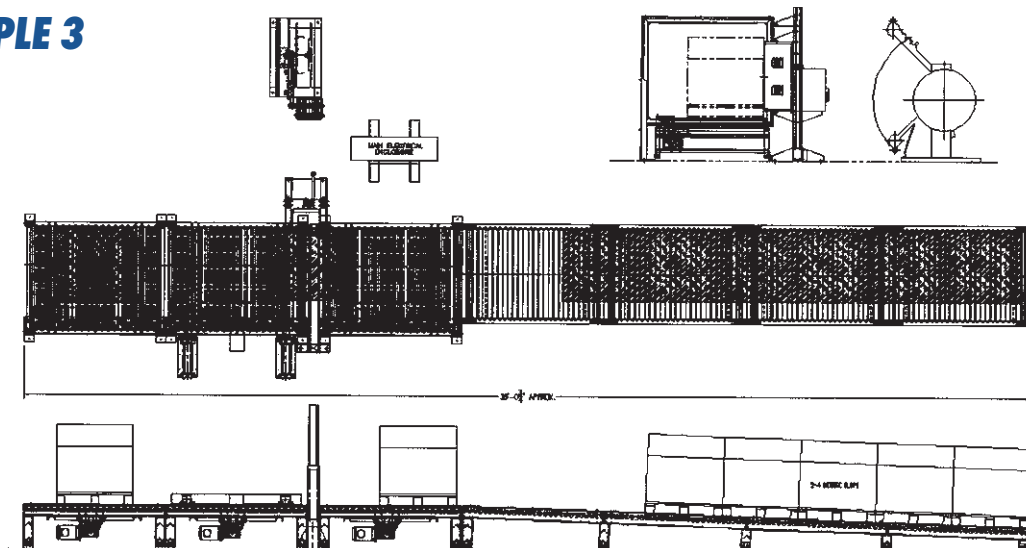
Stand Alone Mini System 2x0 Strap Pattern
